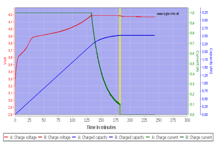
Charakterystyka ładowania akumulatora XTAR 18650 3500mAh
