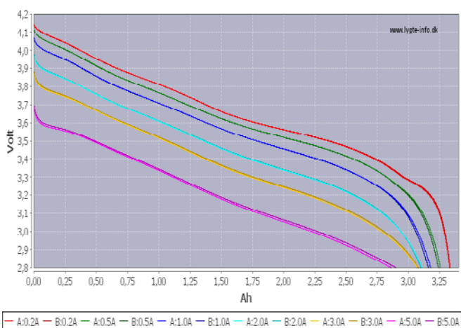
Charakterystyka rozładowania akumulatora XTAR 18650 3500mAh
